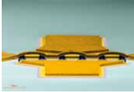
Der neu entwickelte Aluminium-Indiumnitrid-Transistor. (Bild: Andreas Alt, ETH Zürich)
